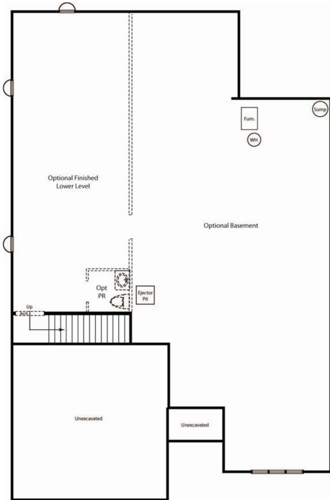
Seville Optional Basement Plan
