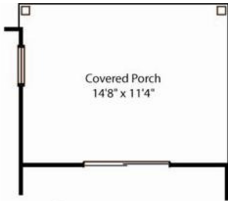
Canaletto Optional Covered Porch
